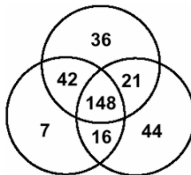
Venn-Diagramm
