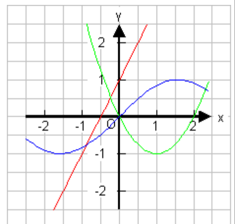
Koordinaten-system
